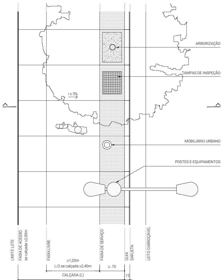
PLANTA
