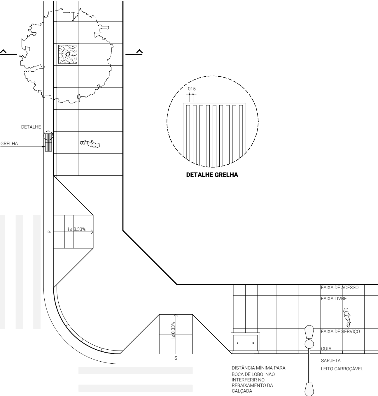
PLANTA
